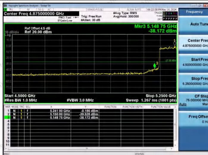
11AX80MIMO-Ant1-5210-PASS
