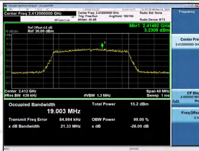
11AX20MIMO-Ant2-2412
