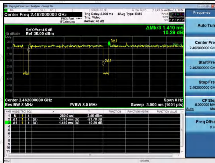
NTNV-11N20MIMO-Ant1-2462
