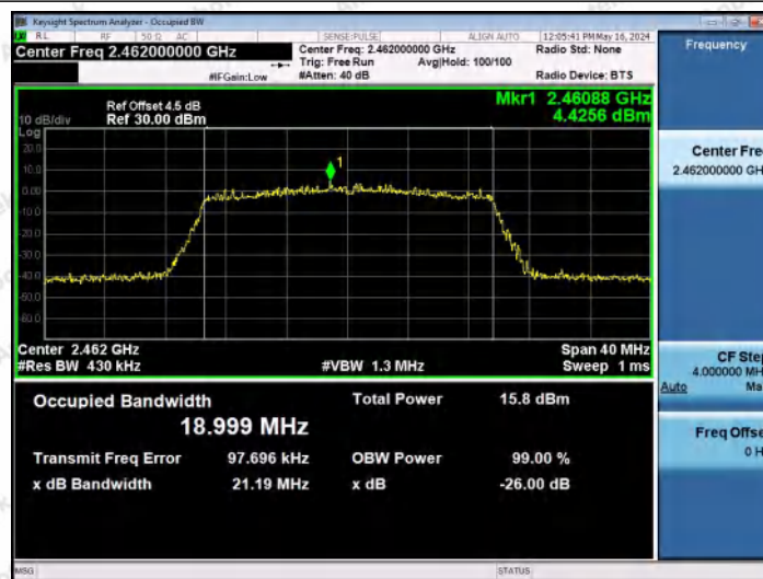
11AX20MIMO-Ant1-2462
