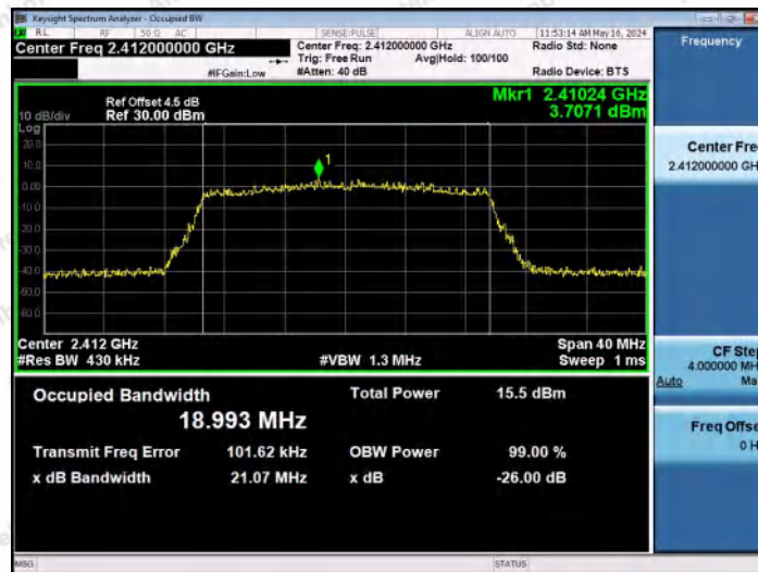
11AX20MIMO-Ant1-2412
