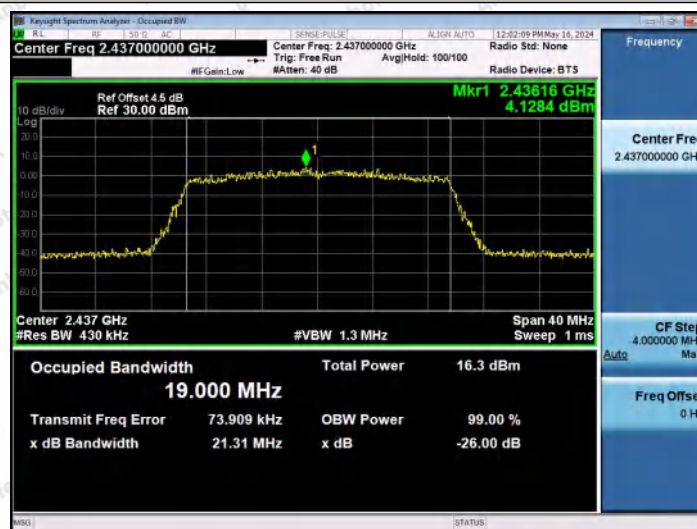
11AX20MIMO-Ant1-2437
