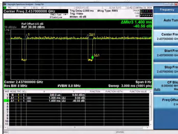
NTNV-11N20MIMO-Ant2-2437
