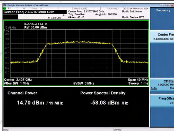
11AX20MIMO-Ant1-2437-PASS
