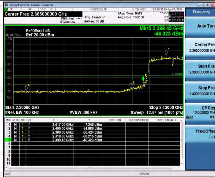
11N40SISO_Ant2_Low_2422
