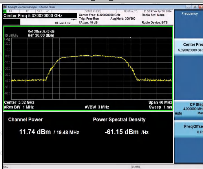
11A_Ant2_5320
