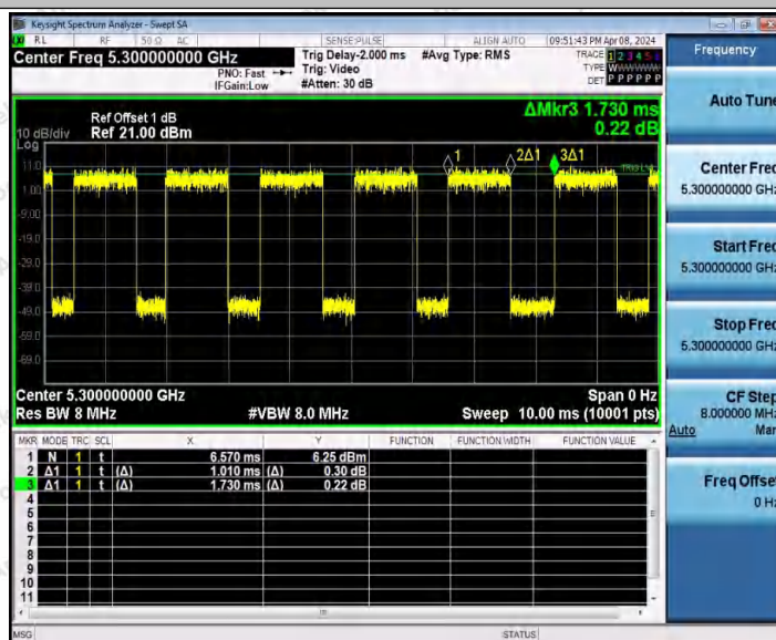
11AX20MIMO_Ant2_5300
