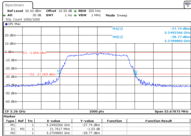
802.11ac20_5260MHz
