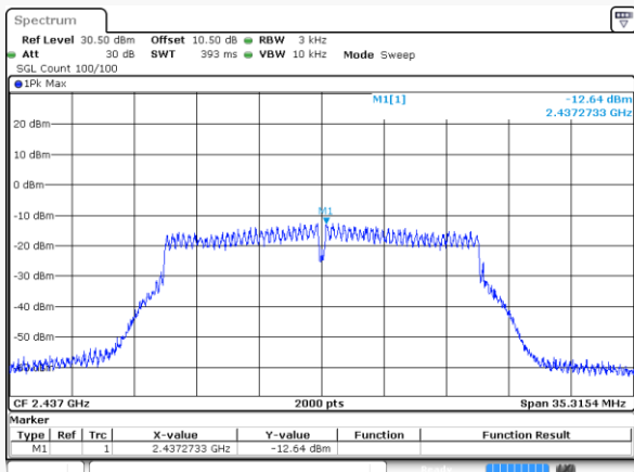
802.11n20_2437MHz_Chain 0
