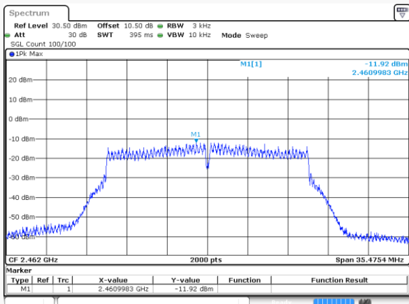
802.11n20_2462MHz_Chain 1
