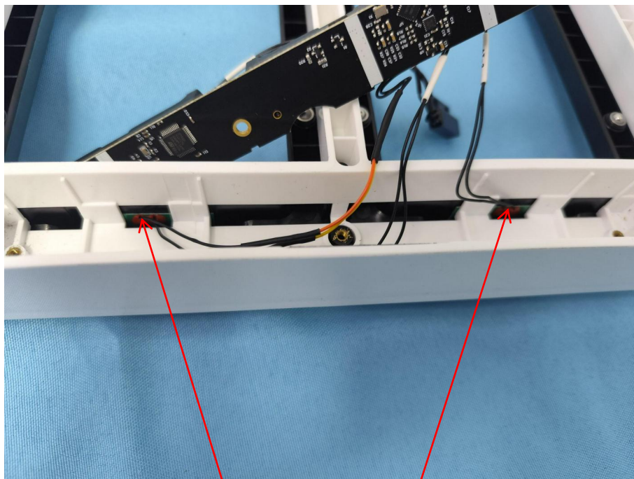
TX ANT1
