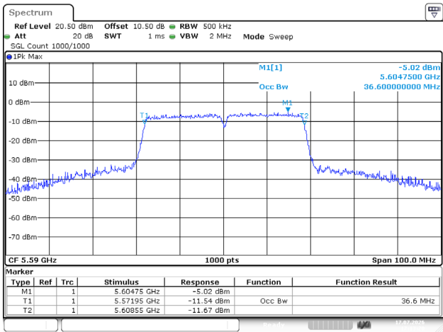
802.11ac40_5590MHz_Chain 1
