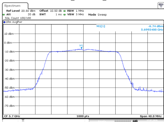
802.11ac20_5700MHz_Chain 1
