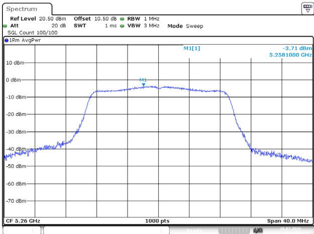
802.11ac20_5260MHz_Chain 1
