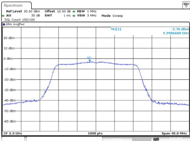
802.11ac20_5300MHz_Chain 0
