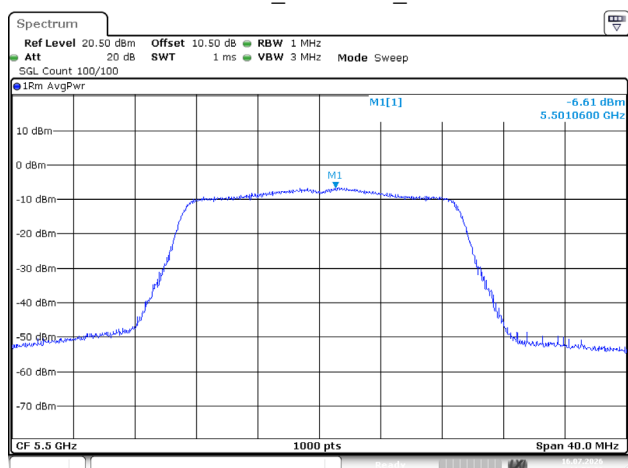
802.11ac20_5500MHz_Chain 0
