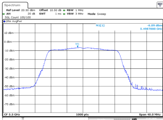
802.11ac20_5500MHz_Chain 1
