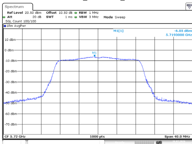
802.11ac20_5720MHz_Chain 0
