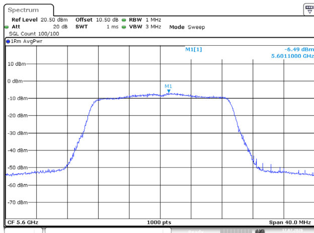
802.11ac20_5600MHz_Chain 1
