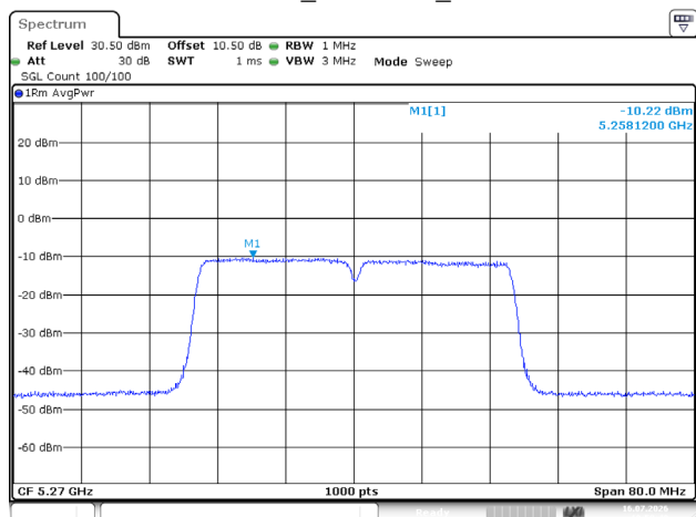
802.11ac40_5270MHz_Chain 0
