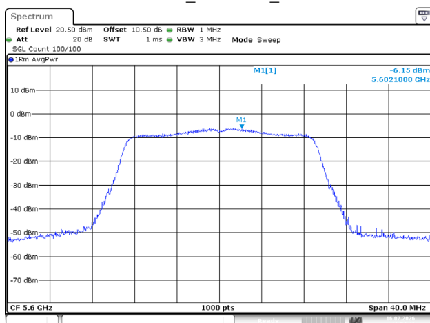
802.11ac20_5600MHz_Chain 0
