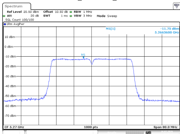
802.11ac40_5270MHz_Chain 1
