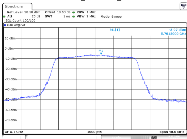
802.11ac20_5700MHz_Chain 0
