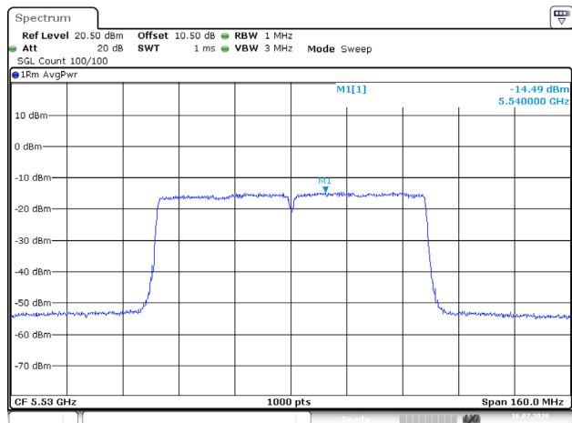
802.11ac80_5530MHz_Chain 0
