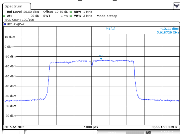
802.11ac80_5610MHz_Chain 1
