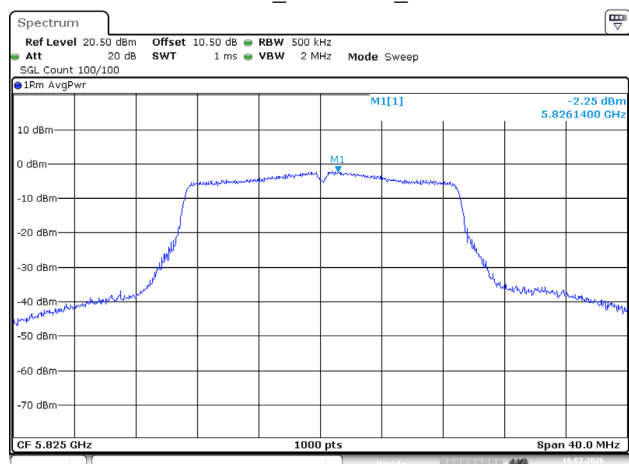
802.11ac20_5825MHz_Chain 0
