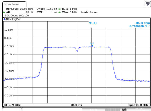
802.11ac40_5710MHz_Chain 0
