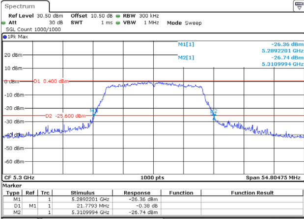
802.11ac20_5300MHz
