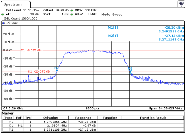
802.11ac20_5260MHz
