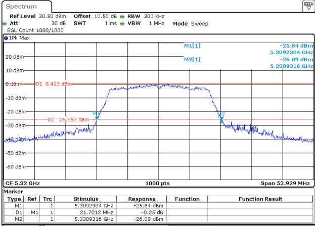
802.11ac20_5320MHz
