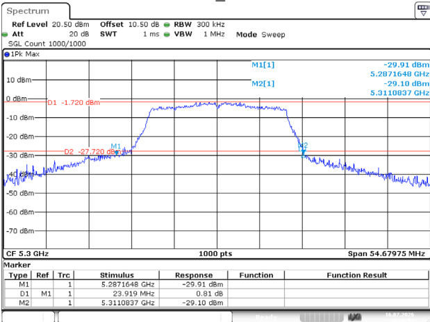
802.11ac20_5300MHz
