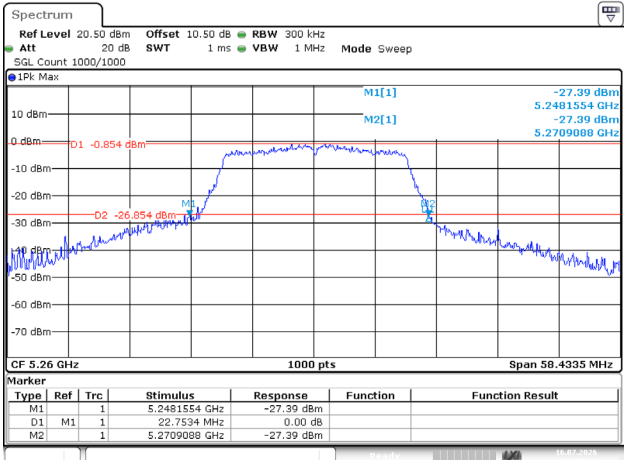
802.11ac20_5260MHz
