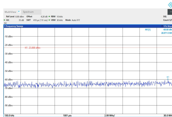
Band2-20MHz-QPSK-18700-1RB#0-Range2:0.15~30MHz
