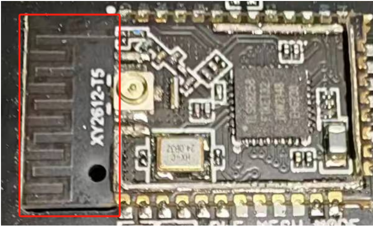
BLE antenna
