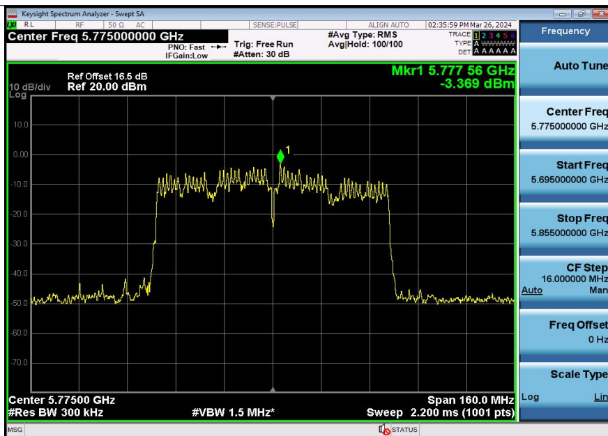
11AC80SISO-Ant1-5775-PASS
