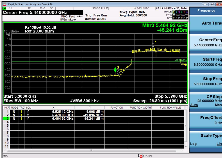
11AX80SISO-Ant3-5530-PASS
