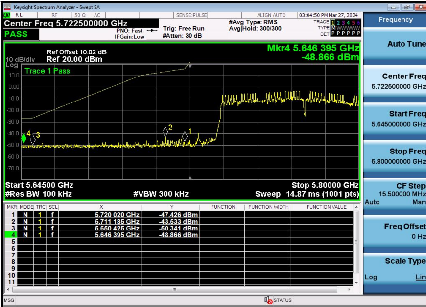
11AC80SISO-Ant3-5775-PASS
