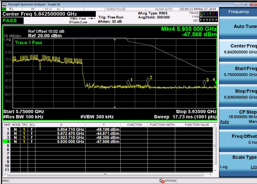
11AC80SISO-Ant3-5775-PASS
