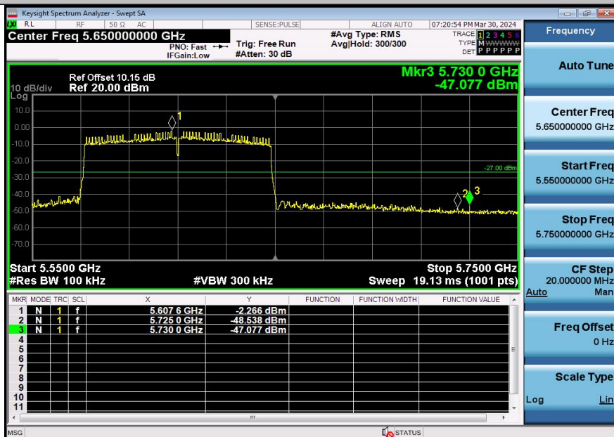
11AX80SISO-Ant3-5610-PASS
