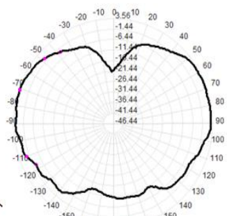
2400.0MHz Total(E1)
