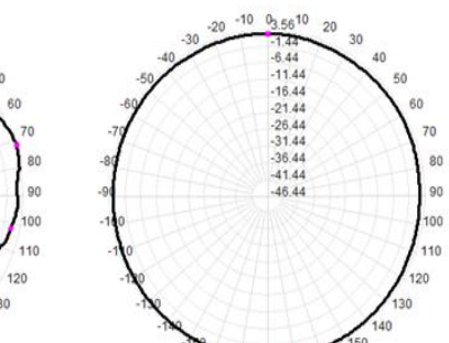
2400.0MHz Total(H)
