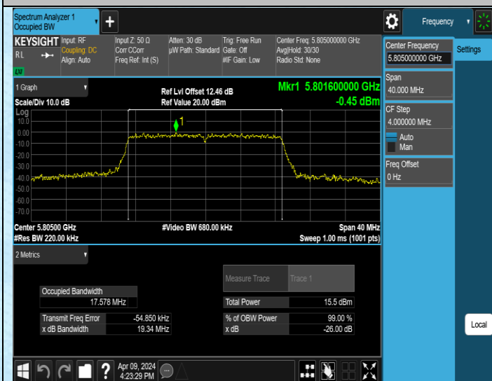
11N20MIMO-Ant3-5805
