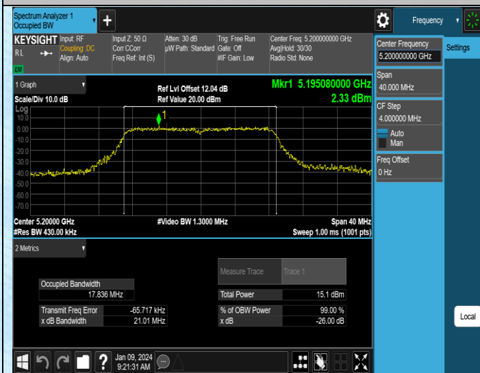
11N20MIMO-Ant3-5200
