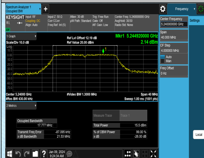
11N20MIMO-Ant3-5240
