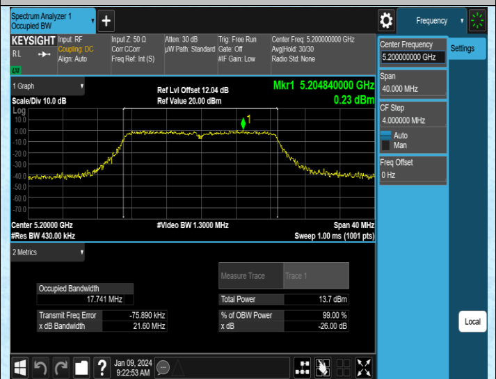
11N20MIMO-Ant4-5200
