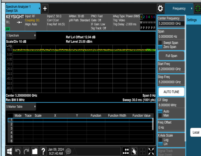
NTNV-11N20MIMO-Ant3-5200
