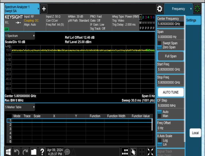
NTNV-11N20MIMO-Ant4-5805
