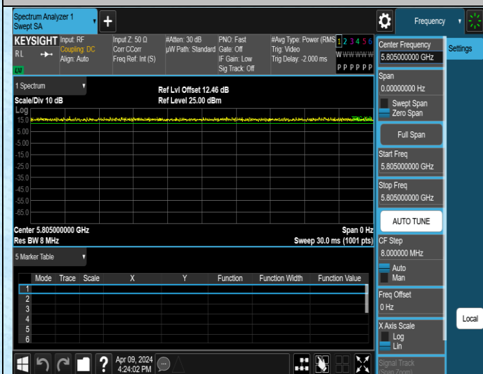
NTNV-11N20MIMO-Ant3-5805
