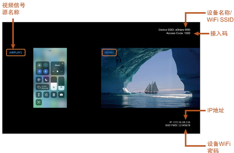
图 3 - OSD 示例二
