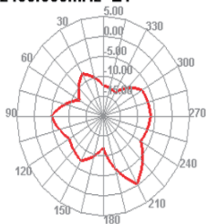
2450.000MHz E1
