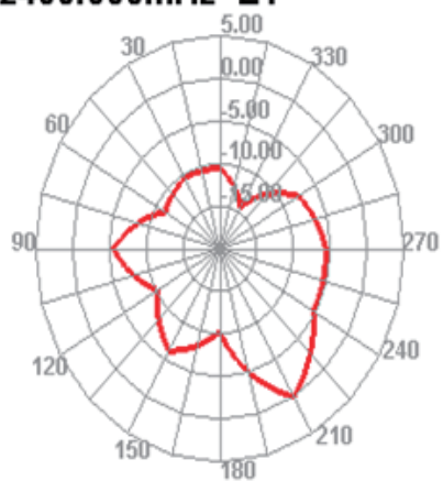
2400.000MHz E1
