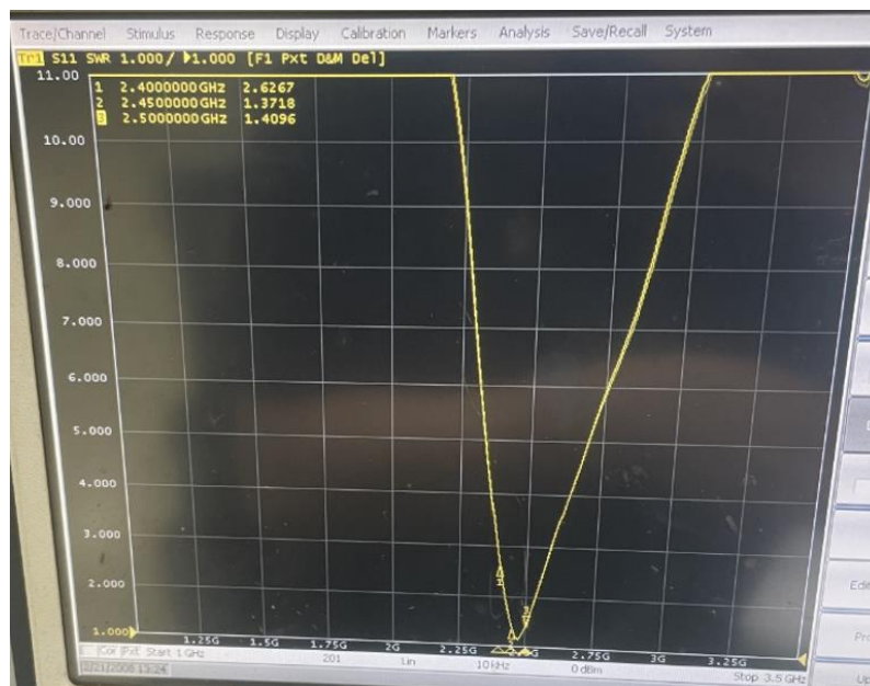
VSWR
