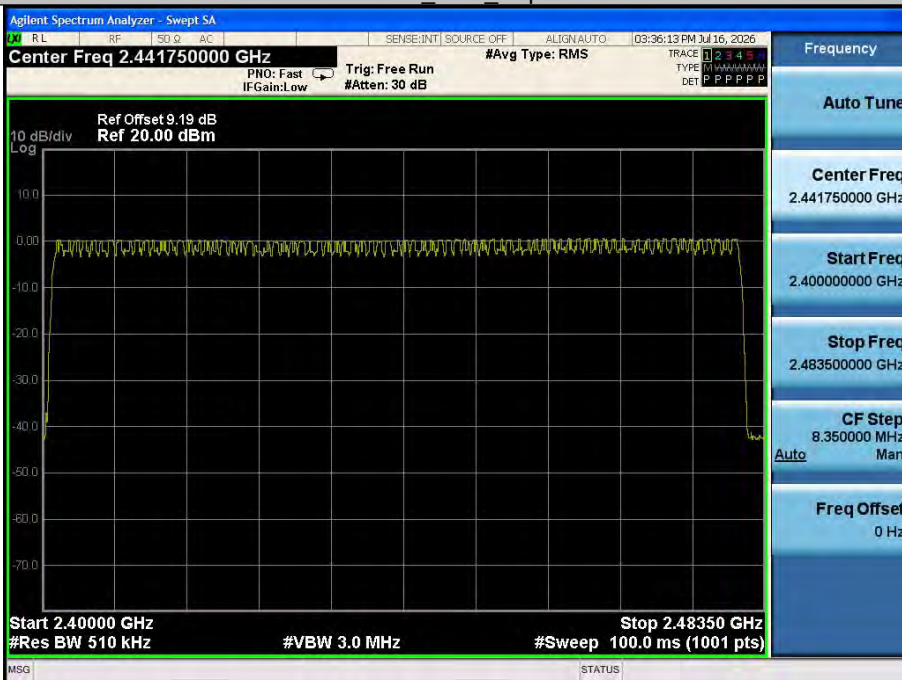
3DH5_Ant1_Hop
