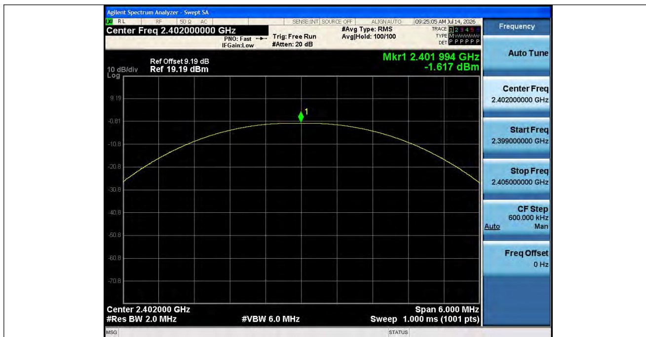
DH5 Ant1 2402
