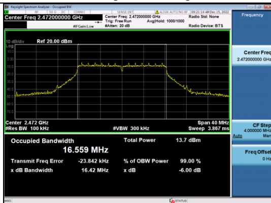
802.11 g / CH 13(High)
