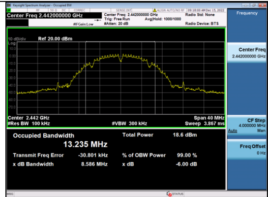
802.11 b / CH 07(Middle)
