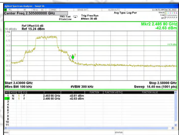
CH11_Ant. 0
