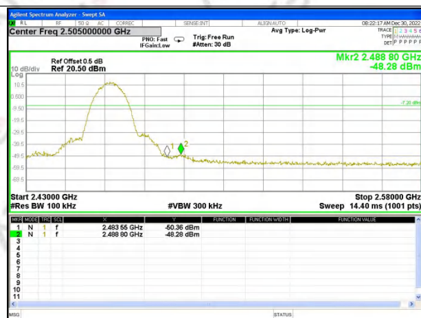
CH11_Ant. 1
