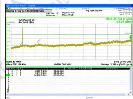
CH3_Ant. 0
