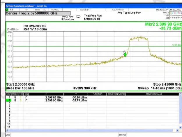
CH1_Ant. 0
