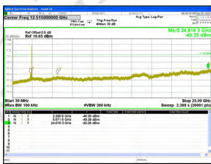
CH6_Ant. 1
