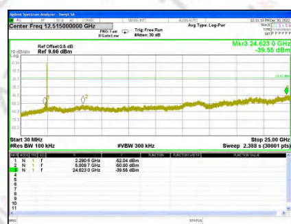
CH9_Ant. 0
