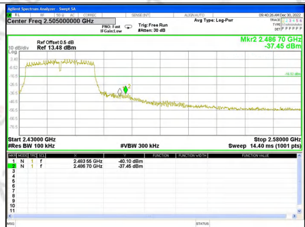
CH9_Ant. 1
