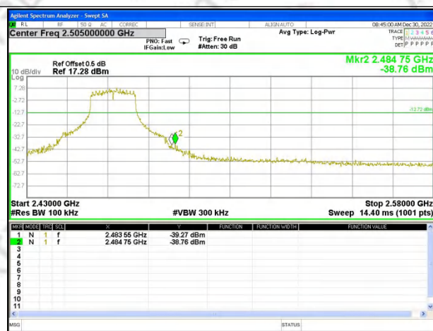
CH11_Ant. 0
