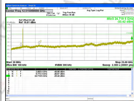
CH3_Ant. 1
