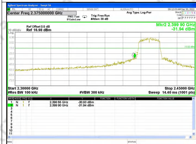
CH1_Ant. 1
