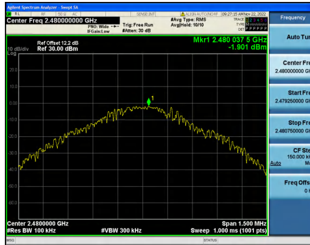
DH5-Ant1-2480-30~1000--1.90
