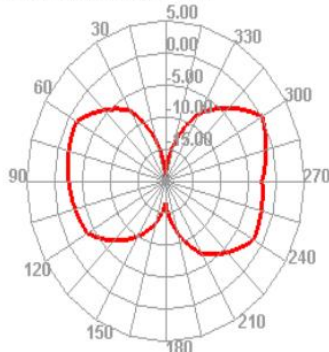
480.000MHz H
