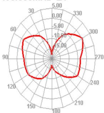
490.000MHz E1
