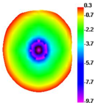
470.000MHz E1
