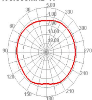
490.000MHz E2
