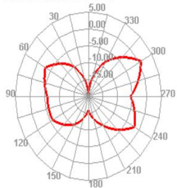
480.000MHz E1
