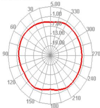
470.000MHz E2
