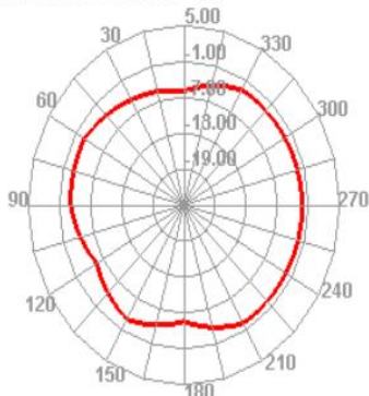
480.000MHz E2
