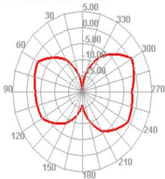
480.000MHz E2
