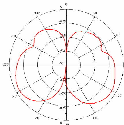
AN2051 E-Plane
