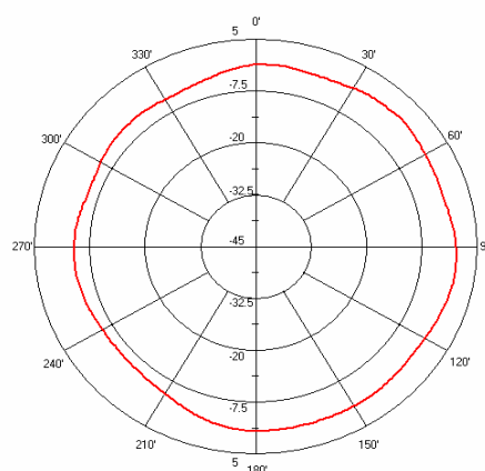
AN2051 E-Plane
