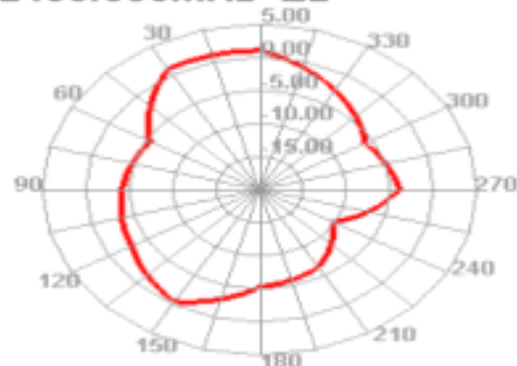
2500.000MHz H
