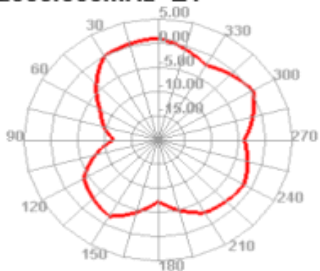
2500.000MHz E1
