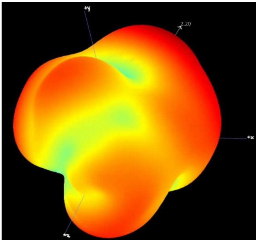
2460MHz 3D
