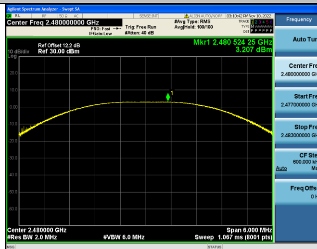
BLE_2M-Ant1-2480
