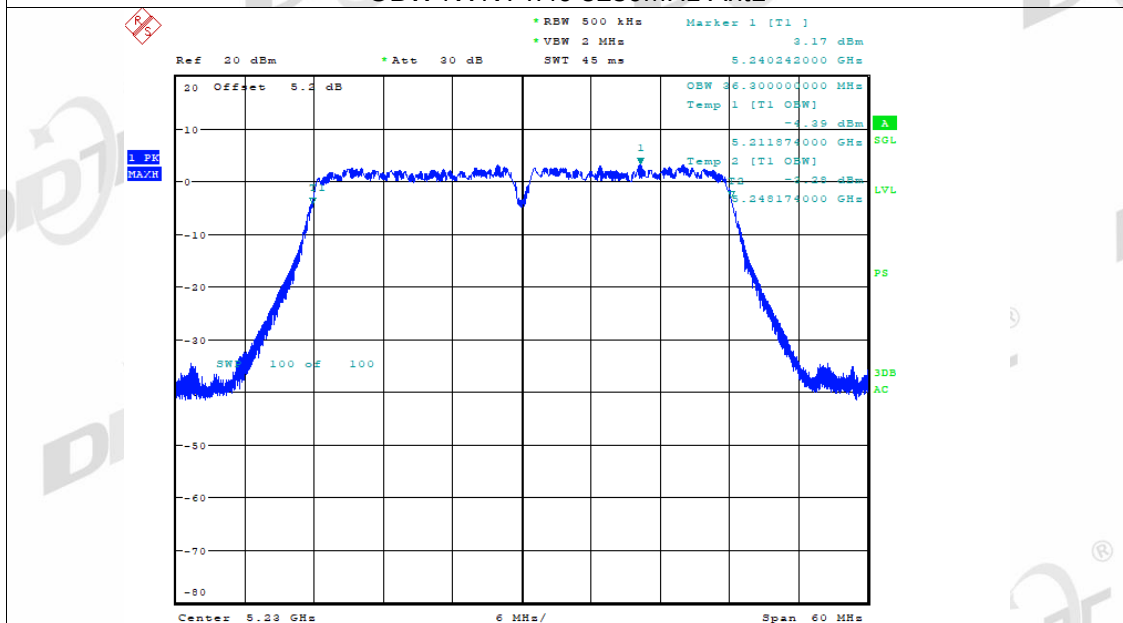
OBW NVNT n40 5230MHz Ant1
