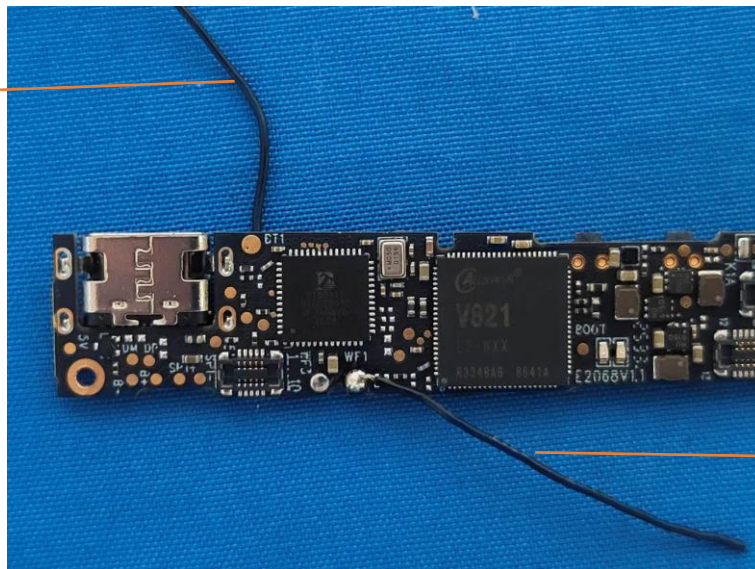
BT ANT
