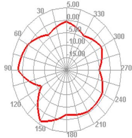
2400.000MHz E2
