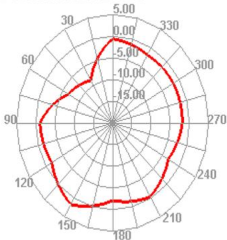
2400.000MHz E1
