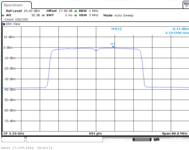
11AX40MIMO-Ant1-5230-PASS
