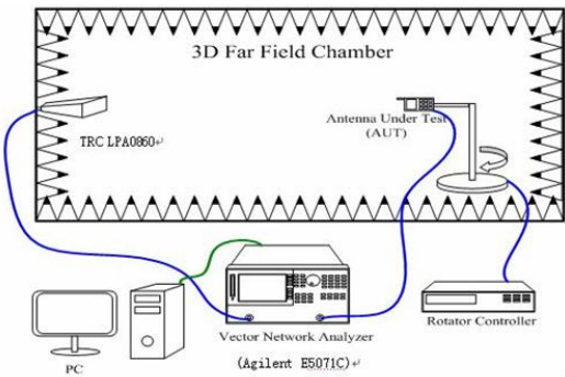
图 1. 微波暗室内部仪器设置
