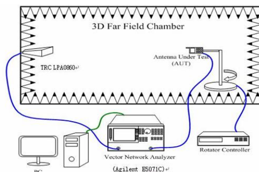
图 1. 微波暗室内仪器设置
