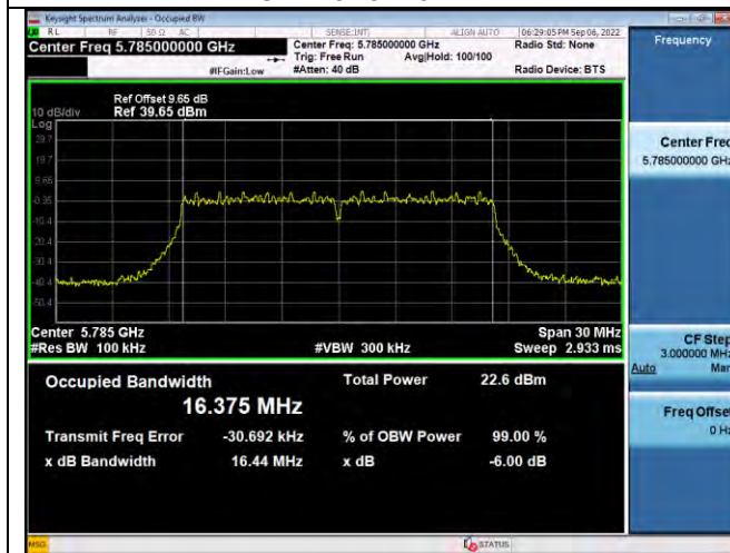
CH157 -5785MHz
