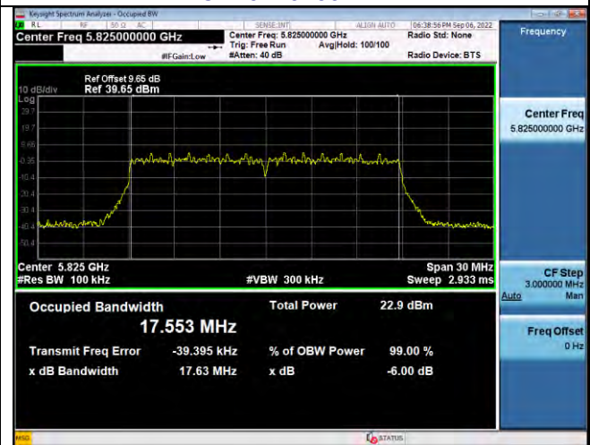
CH165 -5825MHz
