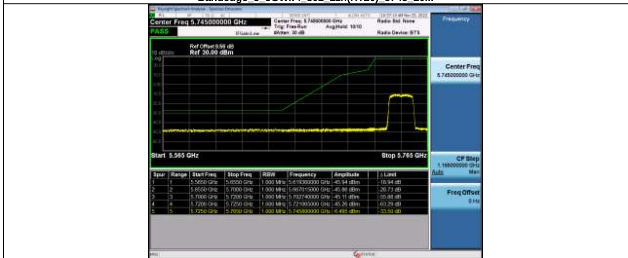
Bandedge 5 8WiFi 802 11n(HT20) 5745 20M
