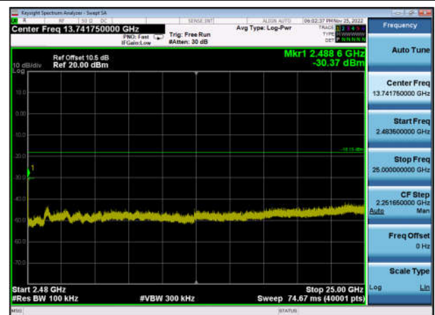
,Plot 4,2483.5MHz~25000MHz-802.11n(HT 40),2452MHz,Ant0
