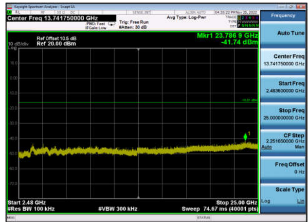
,Plot 4,2483.5MHz~25000MHz-802.11n(HT 20),2462MHz,Ant0
