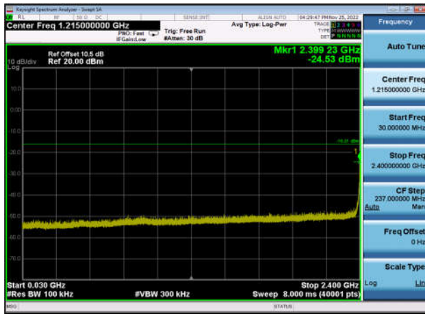
,Plot 3,30MHz~2400MHz-802.11n(HT20), 2462MHz,Ant0
