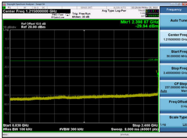
,Plot 3,30MHz~2400MHz-802.11b, 2462MHz ,Ant0
