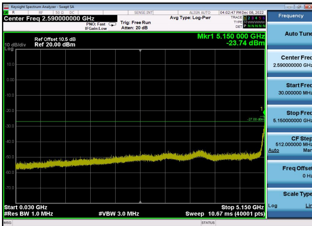
U-NII-1 ,Plot 2,30MHz~5150MHz-802.11a c(80MHz),5210MHz,Ant1
