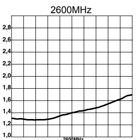
VSWR
