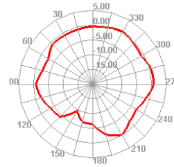
5110.000MHz E2
