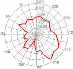
2410.000MHz E1
