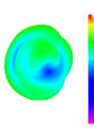
2410.000MHz
