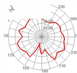
2410.000MHz E2
