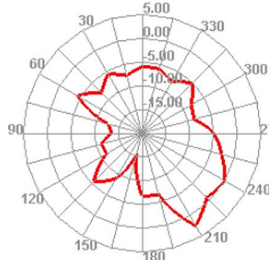
2400.000MHz E1
