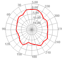
5110.000MHz E1
