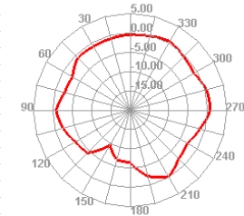
5110.000MHz E2
