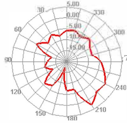
2410.000MHz E1
