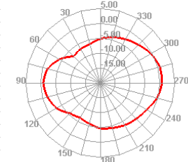
5110.000MHz E2
