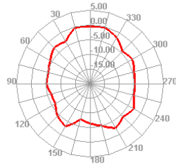
5110.000MHz E1
