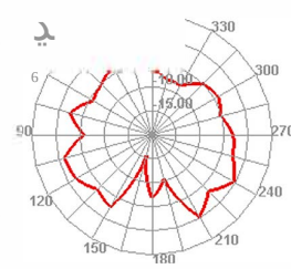
2410.000MHz E2
