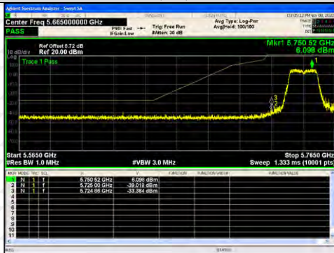
802.11(n40)-5755
