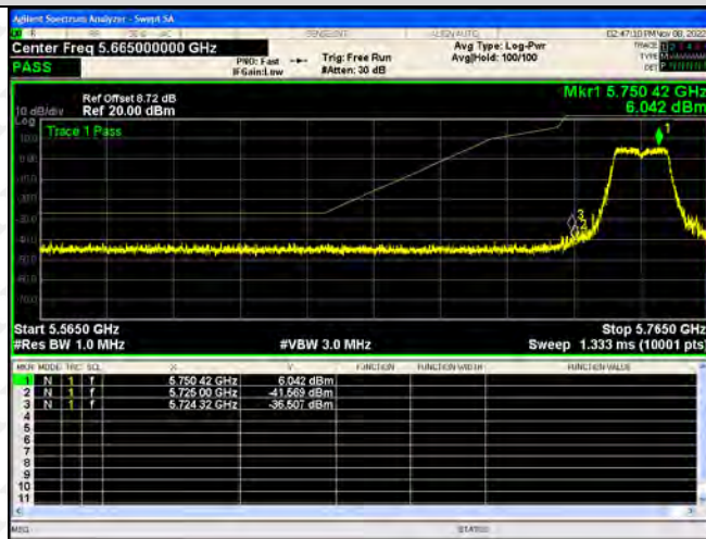
802.11(n20)-5745
