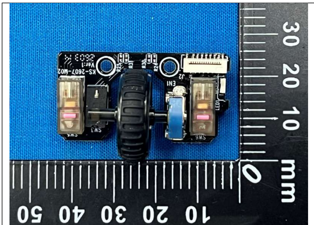
SPDT switch
