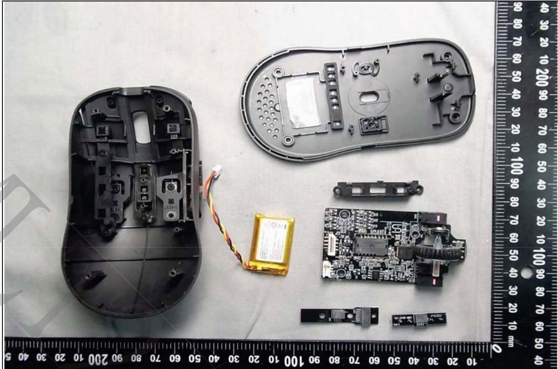
< PCB1-F >
