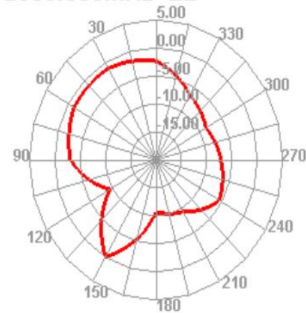
2500.000MHz E2
