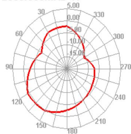
2500.000MHz H
