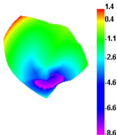
2400.000MHz E1
