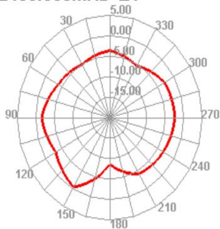
2400.000MHz E1
