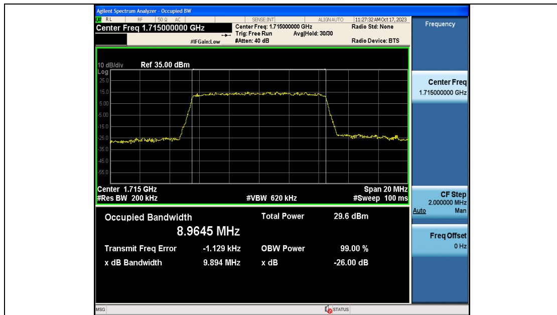
Band4-10MHz-QPSK-20000-50RB#0-PASS
